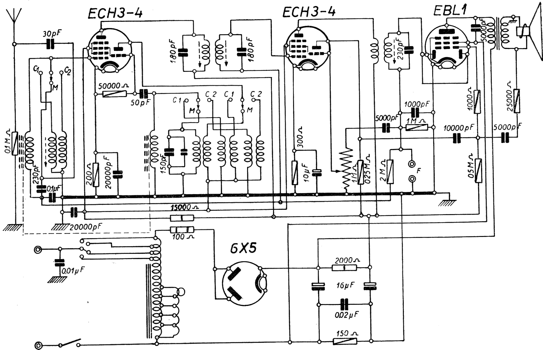
ABC RADIO - Mod. R 841. Supereterodina a variazione di permeabilità, con due induttori variabili. Gamma onde medie da 190 a 590 m, gamme corte da 40 a 50 m e da 24 a 32 m. Media frequenza 465 kc/s. Potenza d'uscita 3 W.
